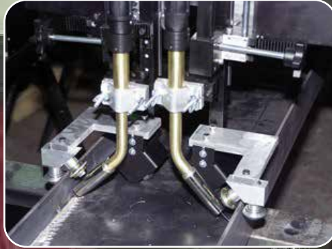
Bug-O Gantry
